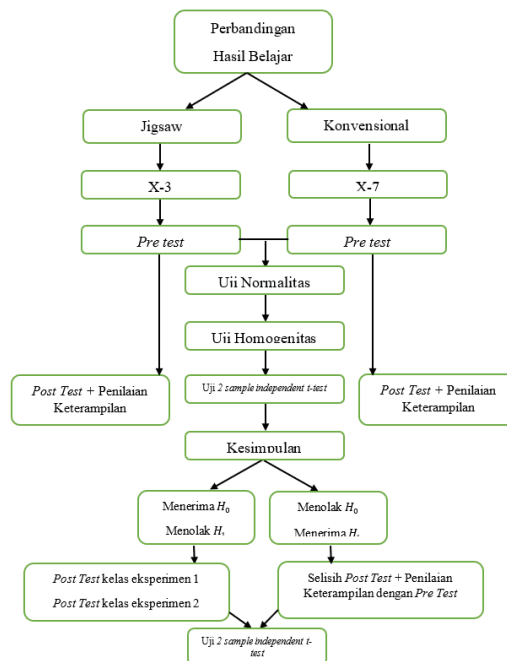
Gambar 1.1 Langkah-langkah Analisis Data Kuantitatif
