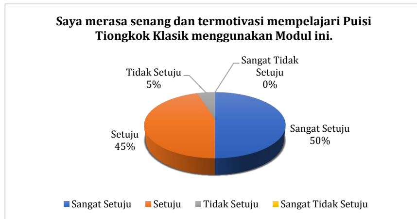
Gambar 2. Persentase responden yang memilih pada pertanyaan pertama
