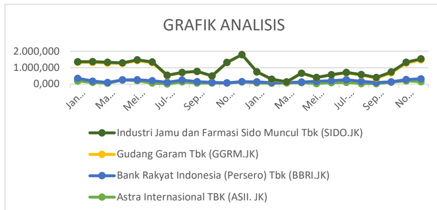
Gambar 1. Grafik Analisis Volalitas Saham
