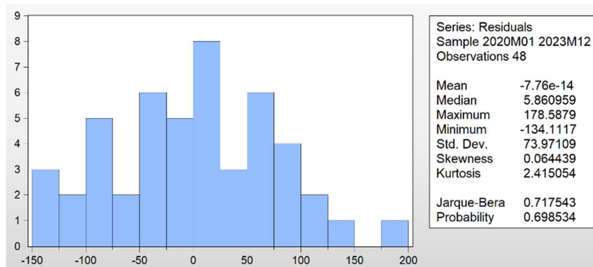
Gambar 3. Uji Normalitas Jarque-Bera.
